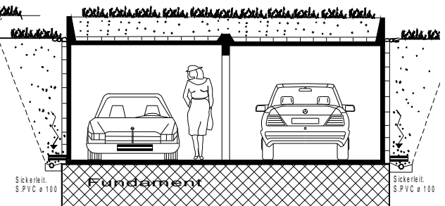
Querschnitt
