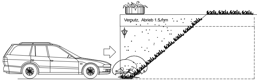
Seitenansicht
