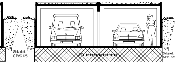
Querschnitt
