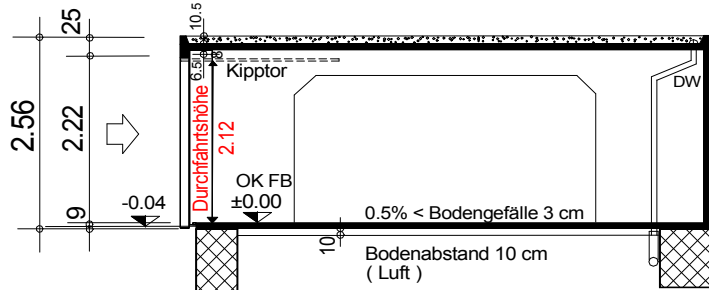
Längsschnitt
