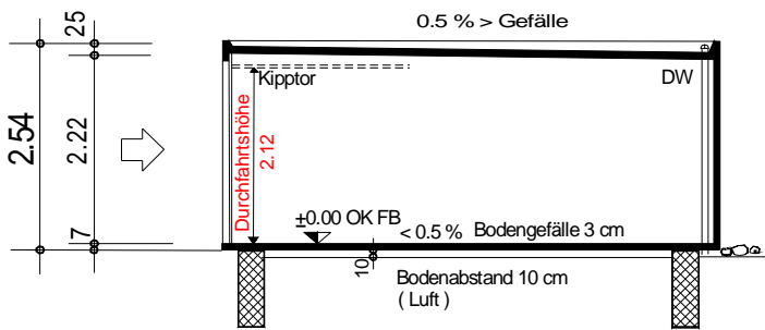
Längsschnitt
