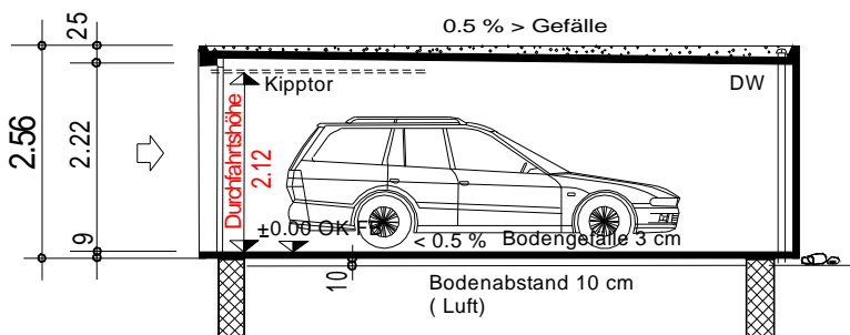
Längsschnitt
