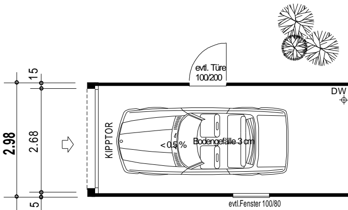
Grundriss
