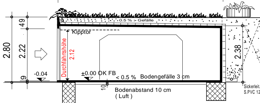
Längsschnitt
