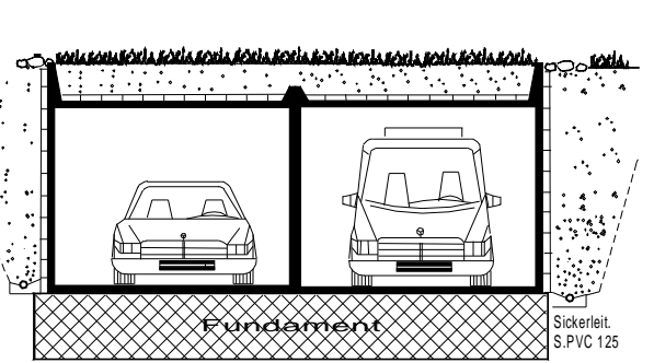
Querschnitt
