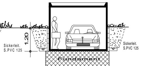
Querschnitt
