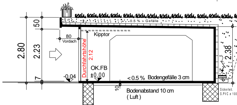
Längsschnitt
